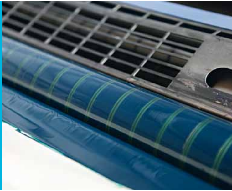
Farbkasten in der Offset-Druckmaschine
